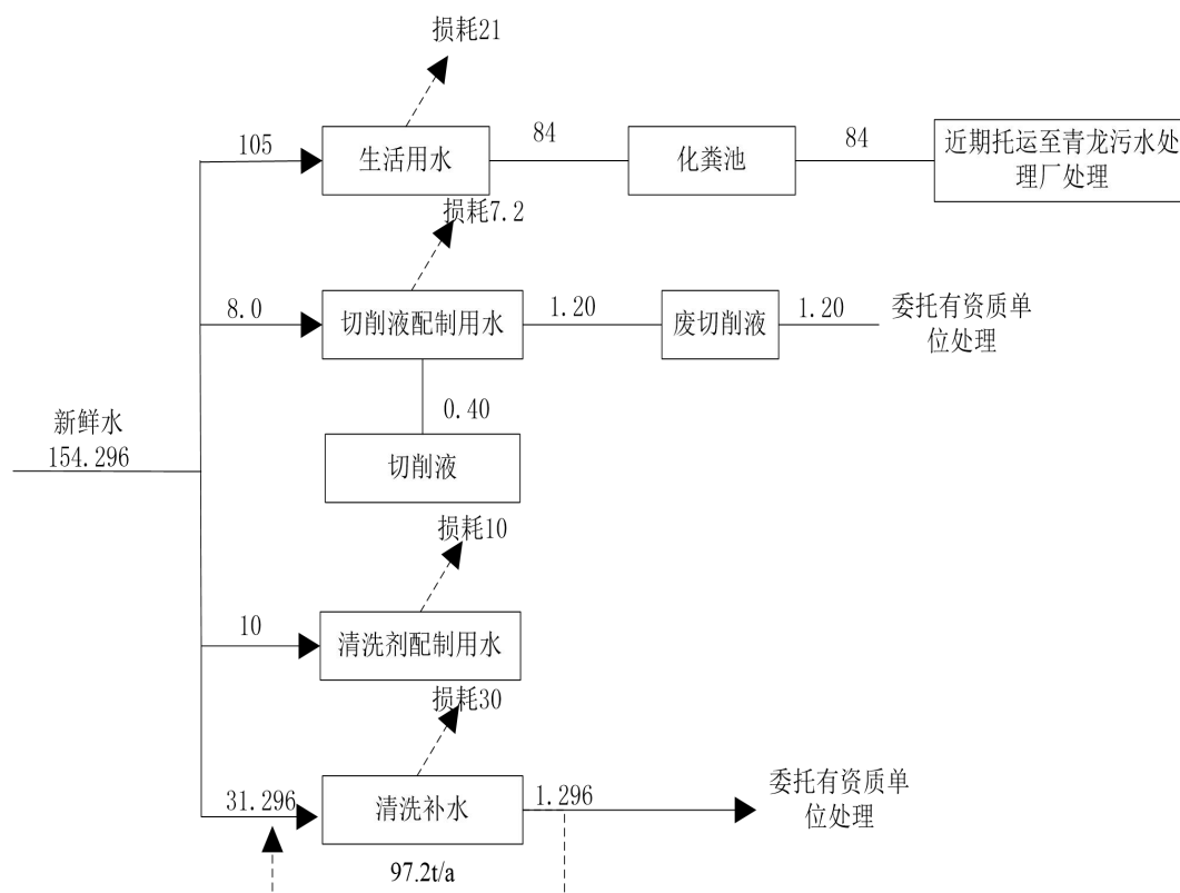
图 5-2 全厂水平衡图(t/a)
