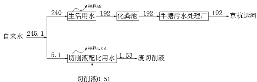
图 5-2 本项目水平衡图 单位：m 3 /a
