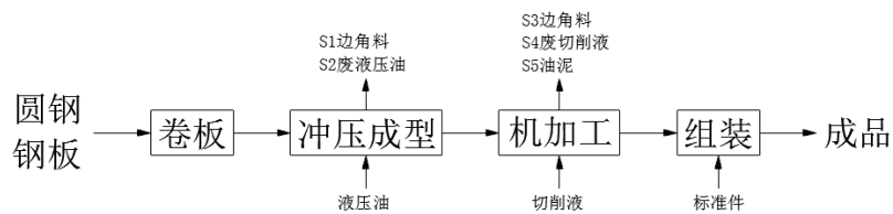
图 5-1 电机零部件制造生产工艺流程及产污环节图
