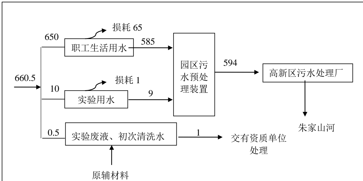
图 2 建设项目水平衡图 (t/a)
