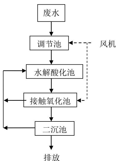
图3 废水预处理工艺流程图
