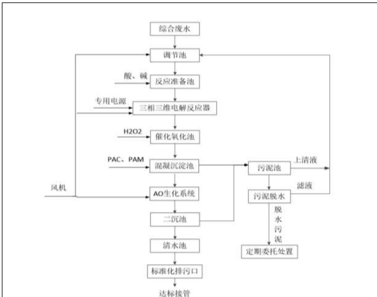
图3 园区废水预处理工艺流程图
