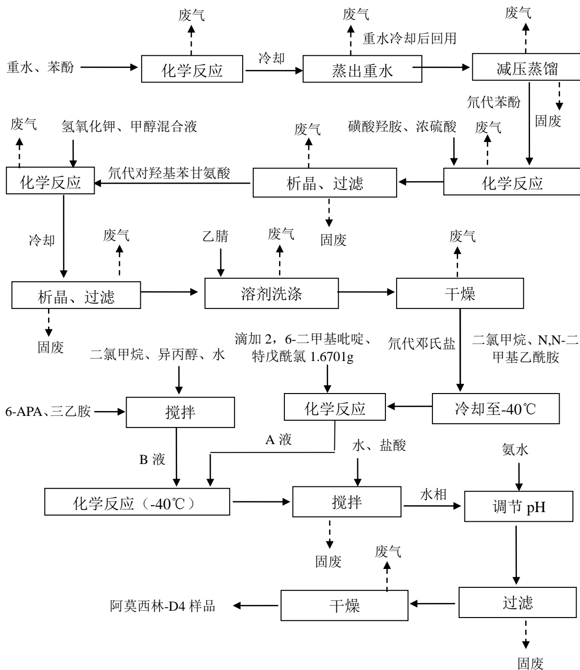
图 1 重水标定阿莫西林工艺流程及产物环节图
