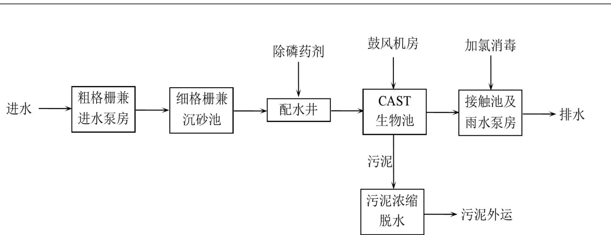
图 3 仙林污水处理厂污水处理工艺流程图
