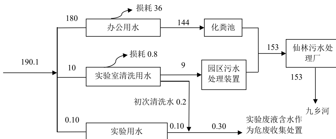
图 3 建设项目用水平衡图 (t/a)
