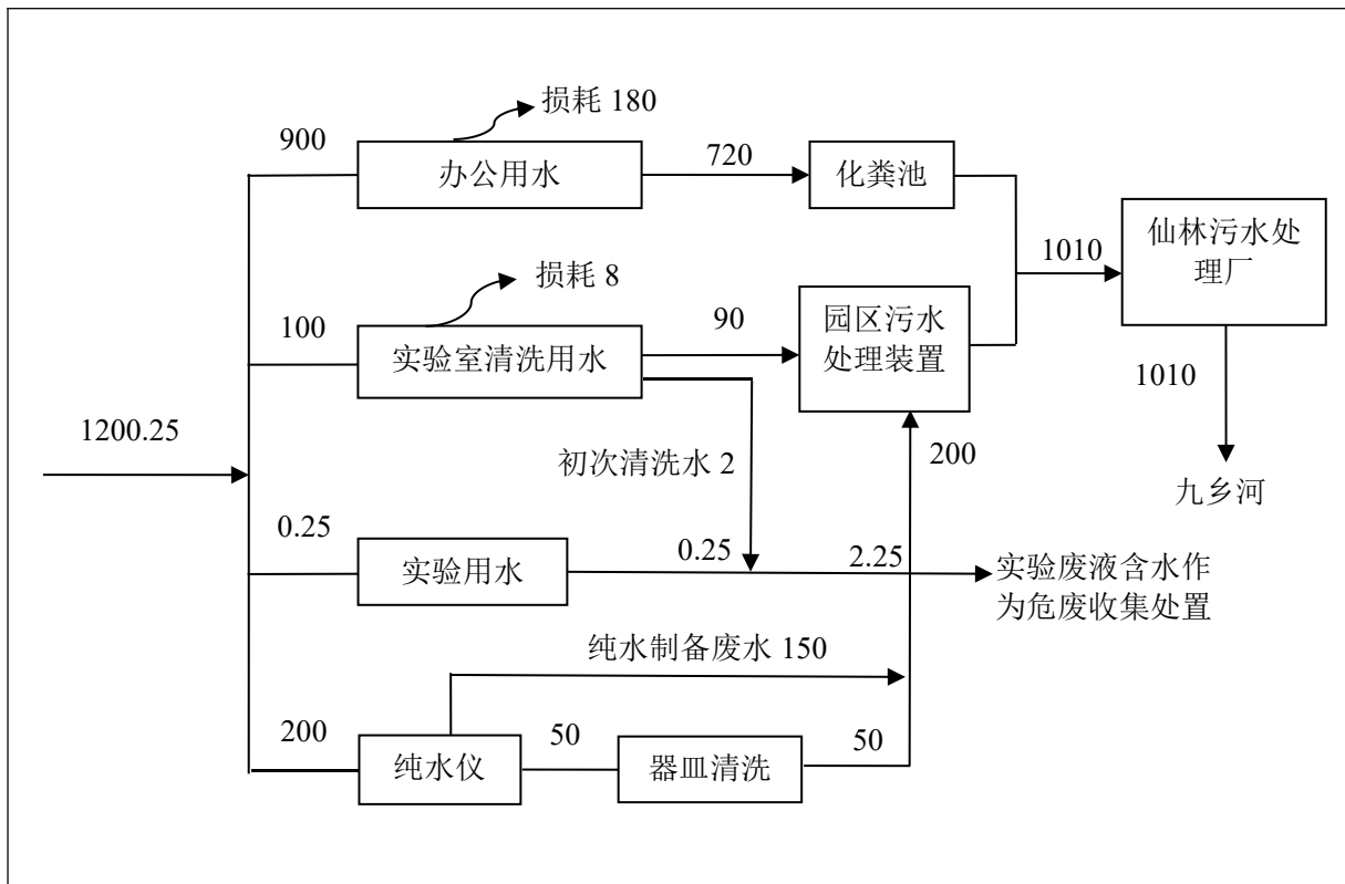
图 3 建设项目用水平衡图 (t/a)
