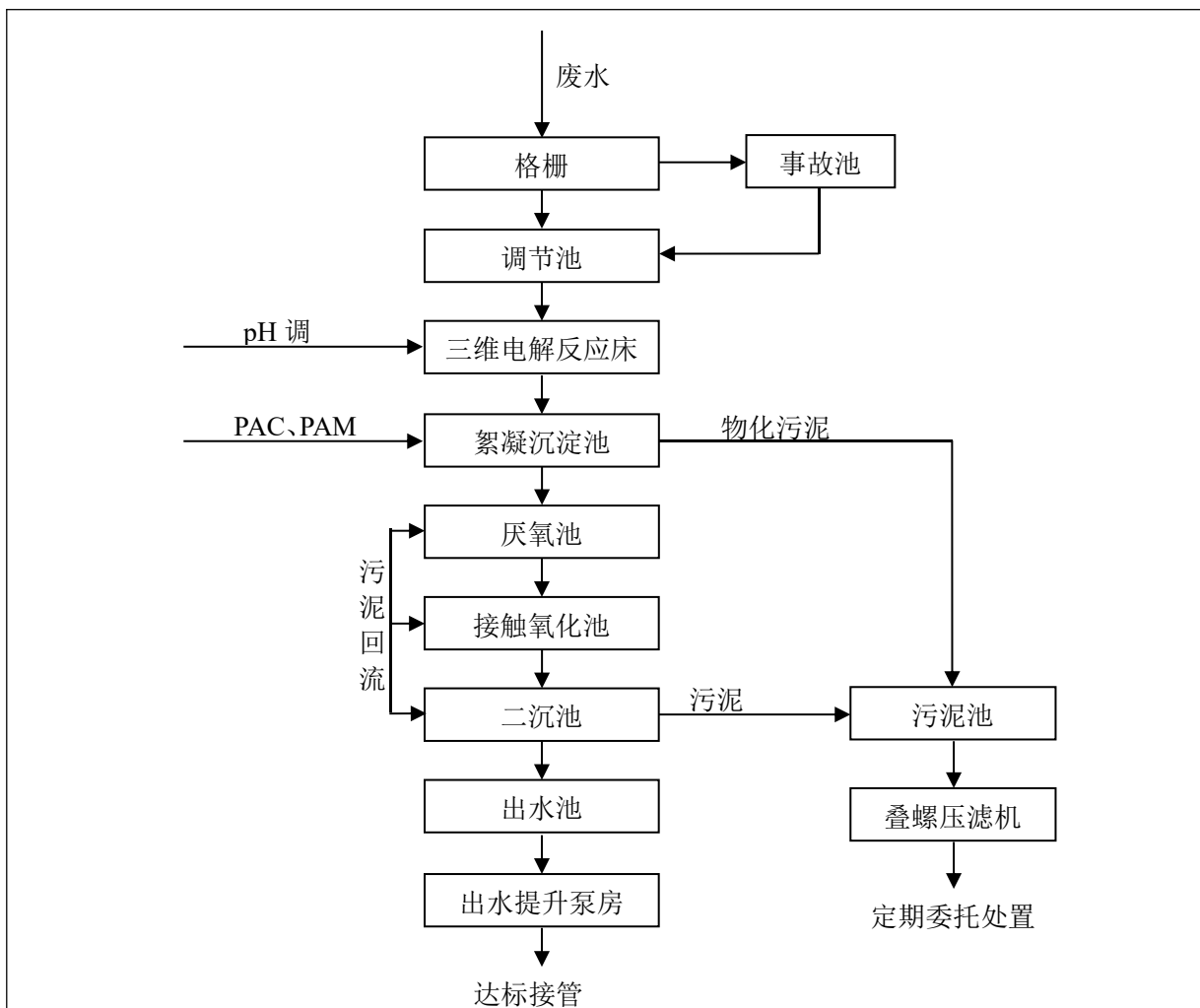
图 2 本项目实验室污水预处理工艺流程图
